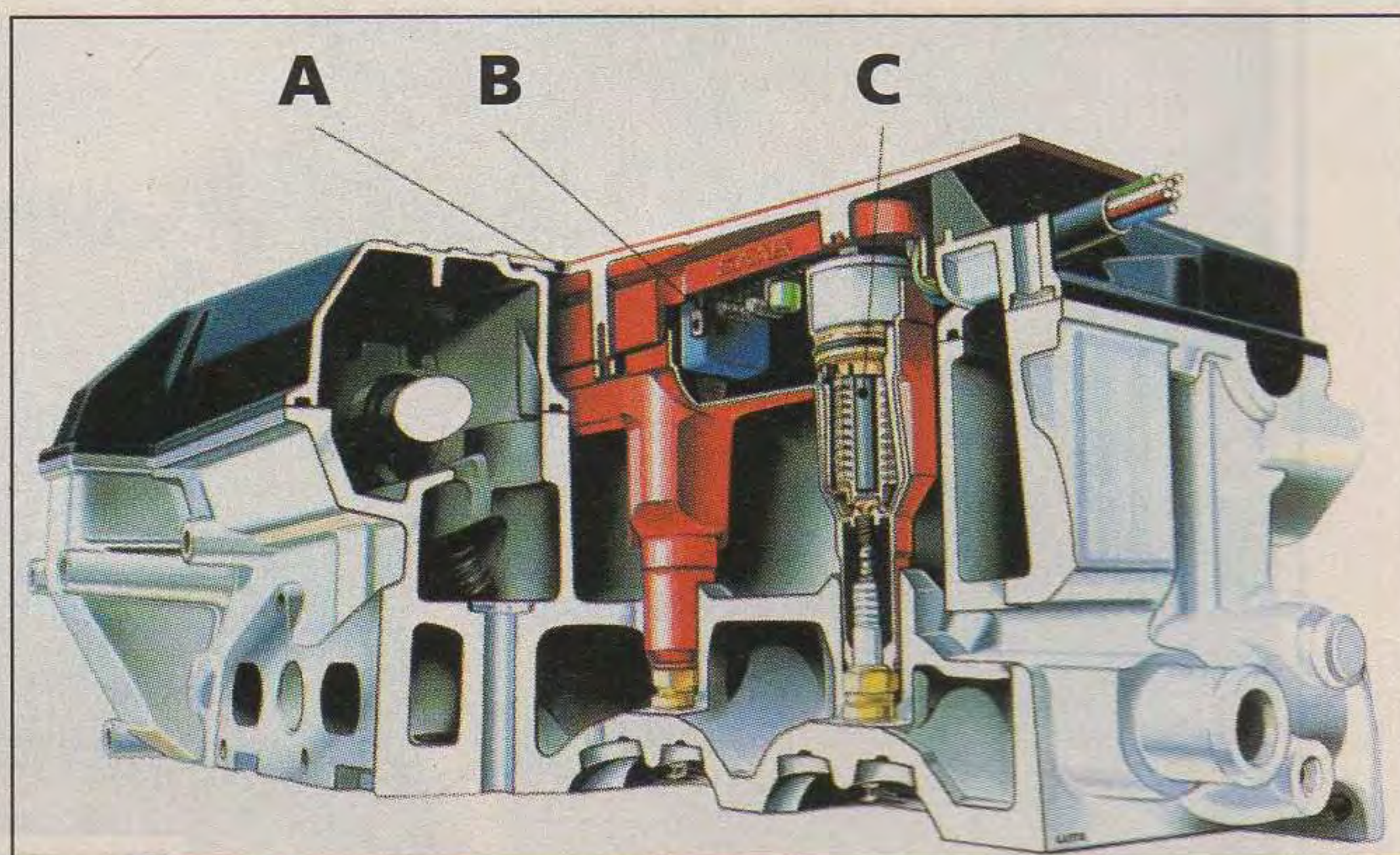
Colocación del sistema de encendido directo Saab SDI en la tapa de cilindros. El cartucho o casete integra a: A) Caja metálica. B) Capacitor. Aumenta el voltaje de 12 a 400 V. C) Una bobina por cilindro. Eleva la tensión de 400 V a 40.000 V.
