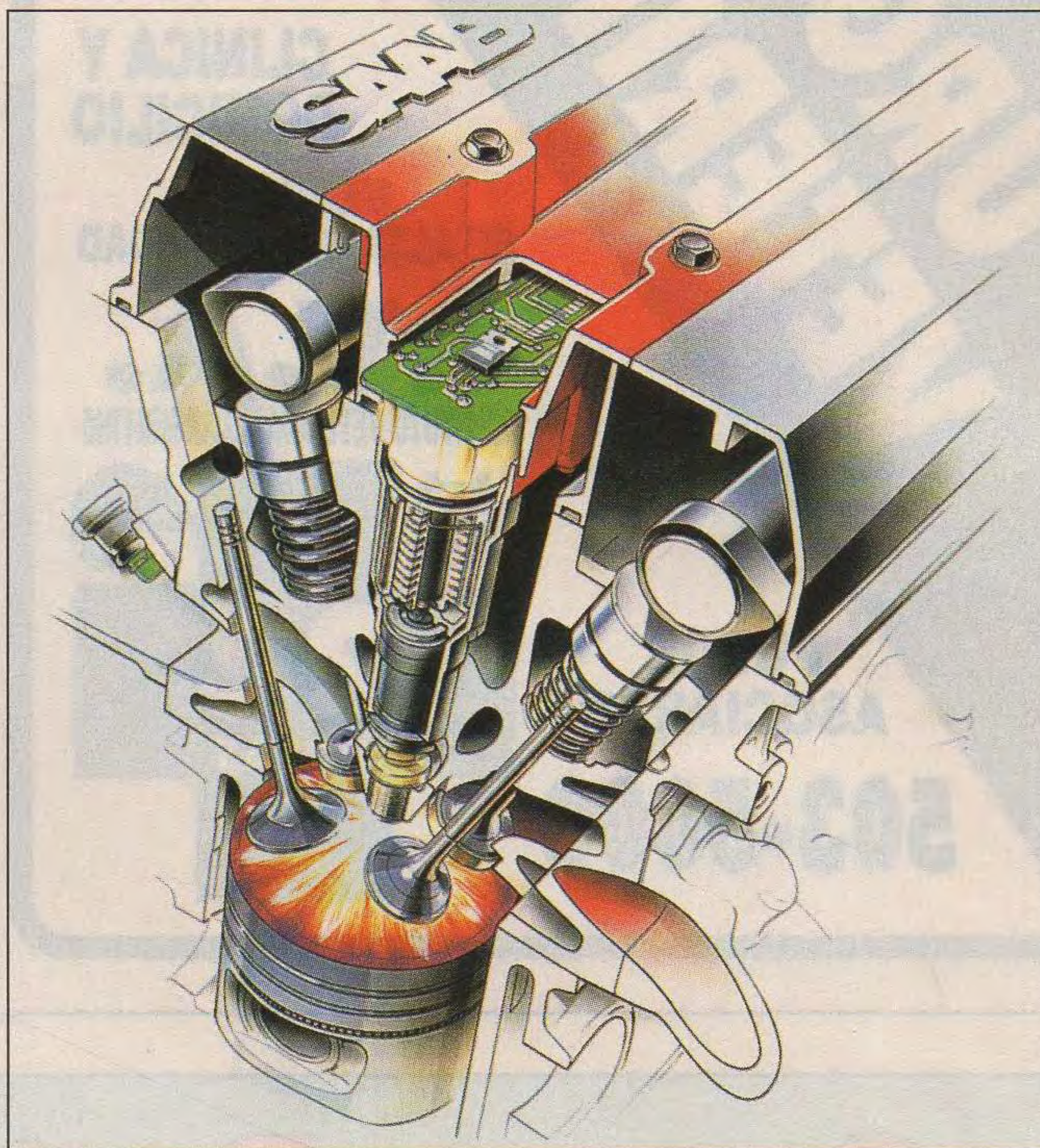
El encendido directo a casete inaugura una nueva era de motores altamente eficientes y poco contaminantes. Nótese la bobina de encendido colocada directamente encima de la bujía y un poco más arriba al circuito electrónico integrado en el casete. Adios a los cables...
