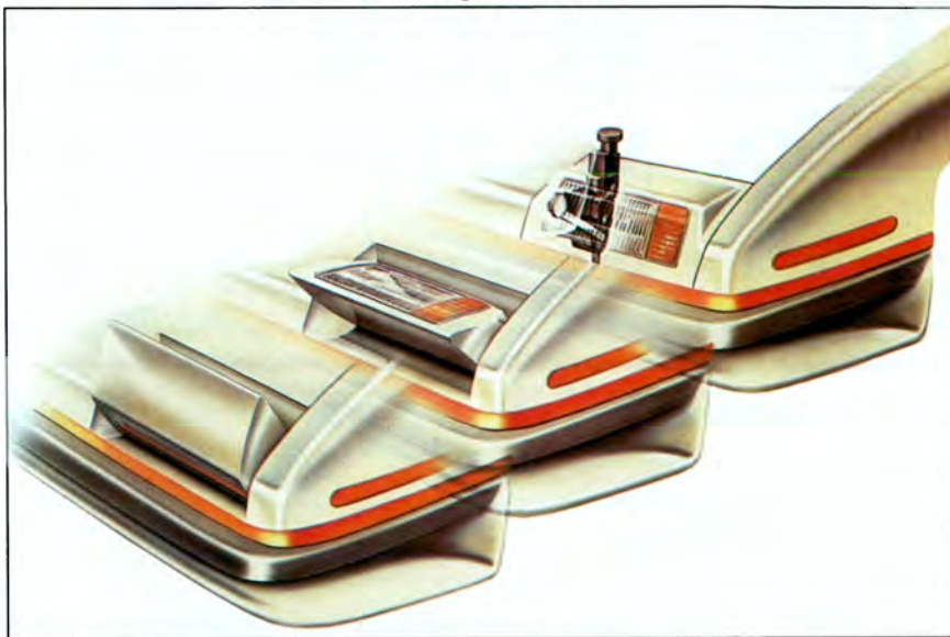
Unidad de faros retráctiles de comando motorizado y de control por microprocesador.
