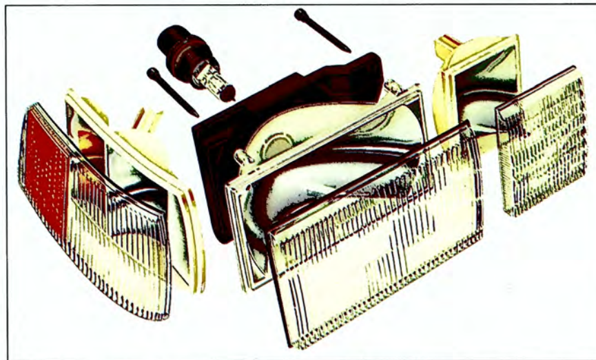
Los cristales de los faros modernos son ahora de policarbonato, más liviano y resistente que el vidrio.
